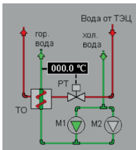
Рис. 13. Пример автоматизированной системы подогрева воды
